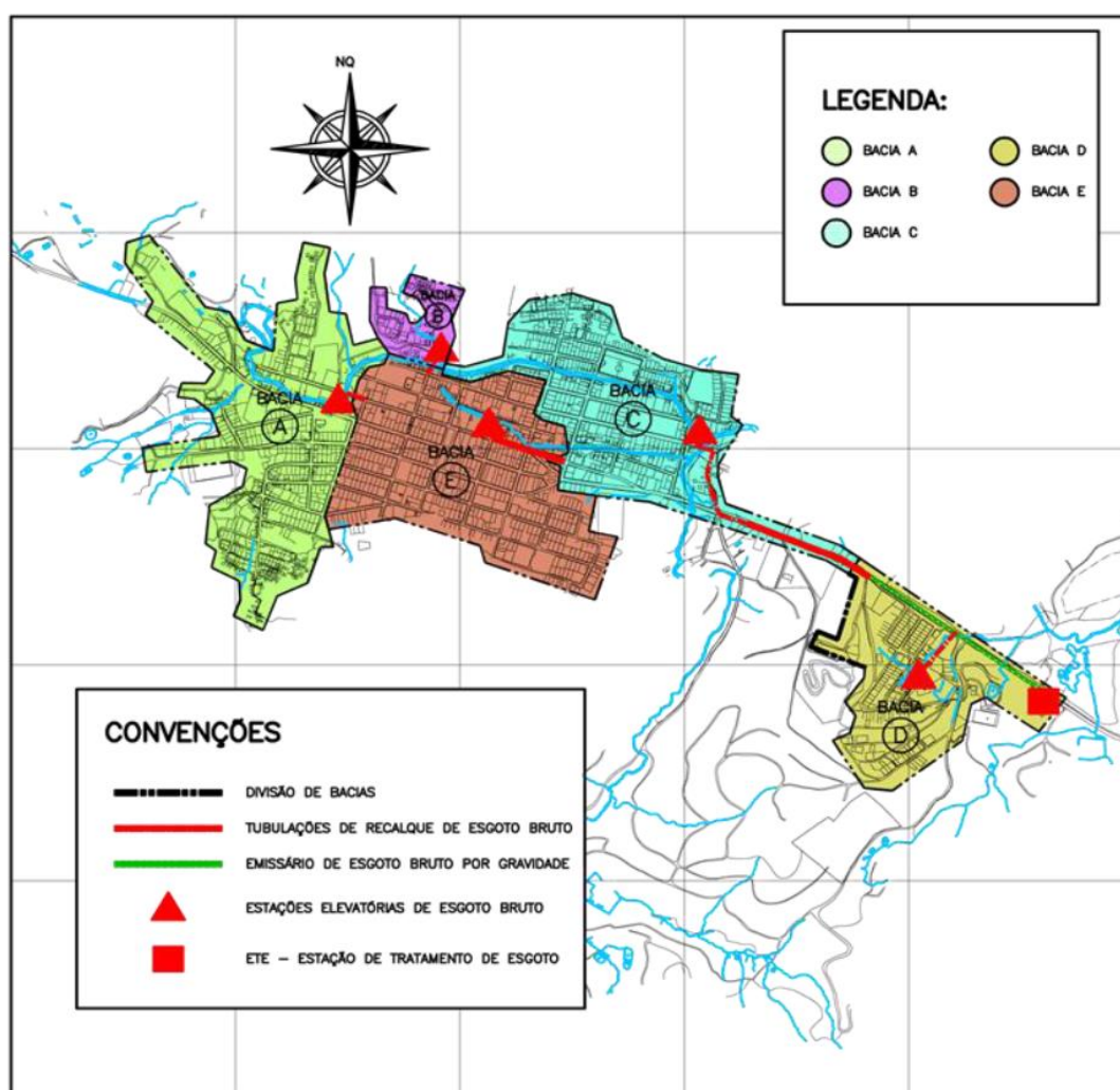
Figura 3-20: Planta esquemática do SES em Pancas Sede.
